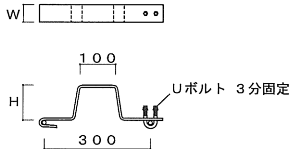
無溶接フープ筋取付型
